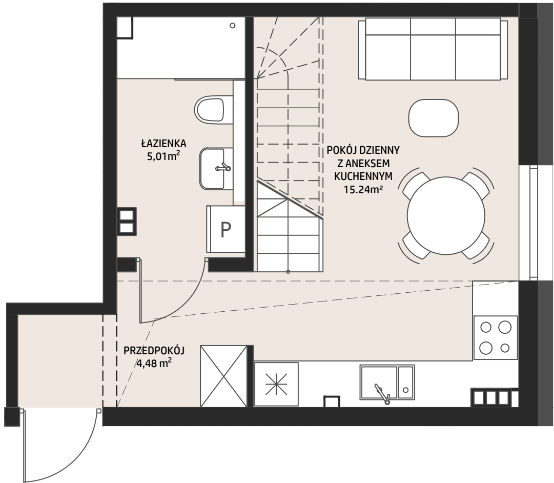
POZIOM 1: 24,73m²
