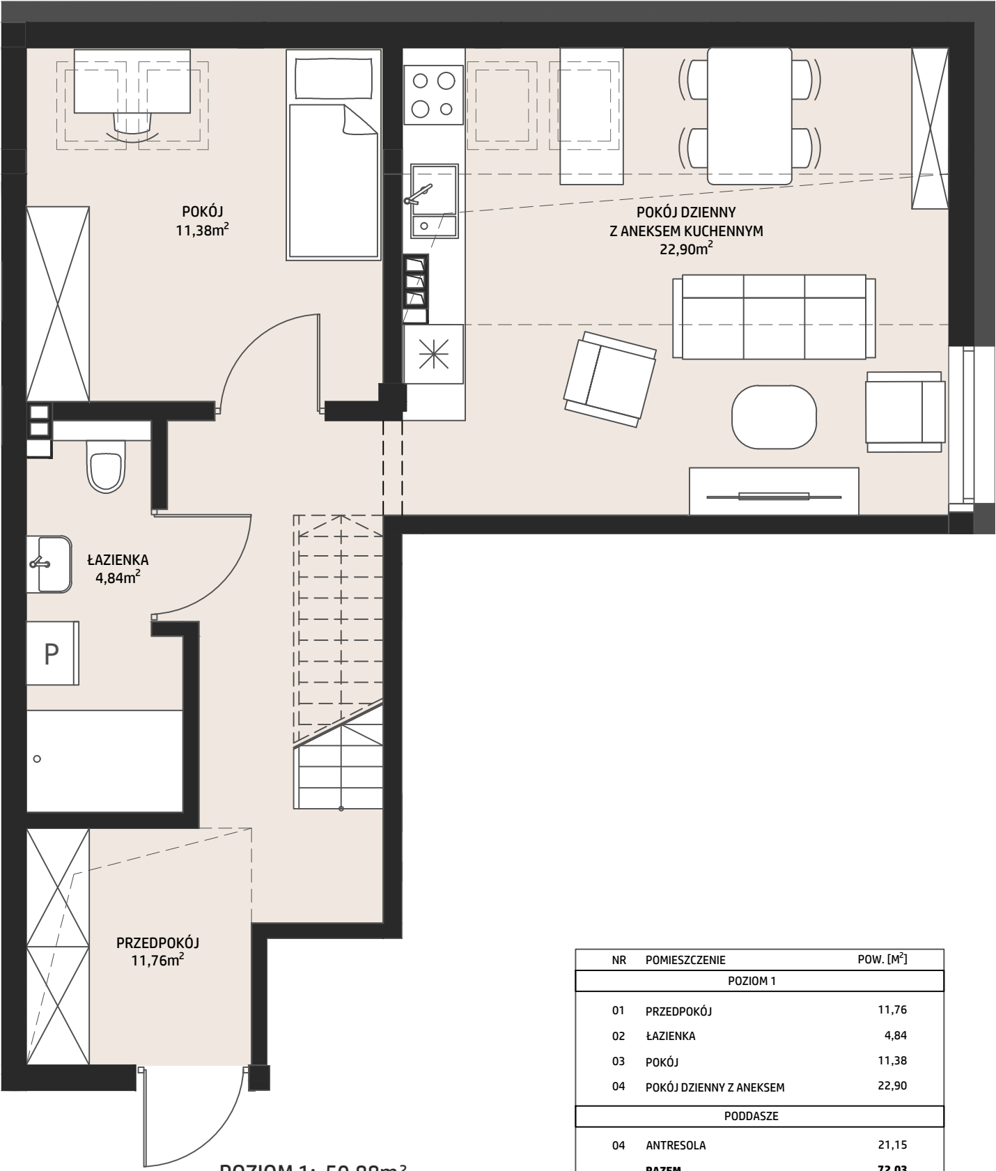
POZIOM 1: 50,88m²
